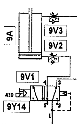
VERIN MAINTIEN MINI CD
