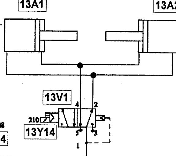
VERIN MAINTIEN MINI CD
