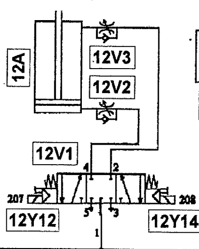
VERIN PRISE BLISTER
