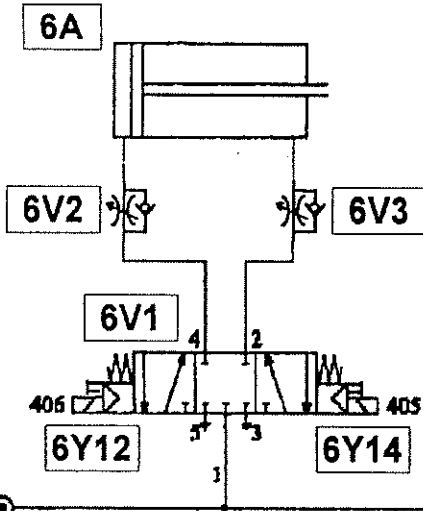
VERIN MAINTIEN BLISTER
