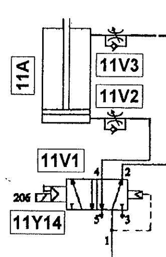
VERIN BUTEE BLISTER
