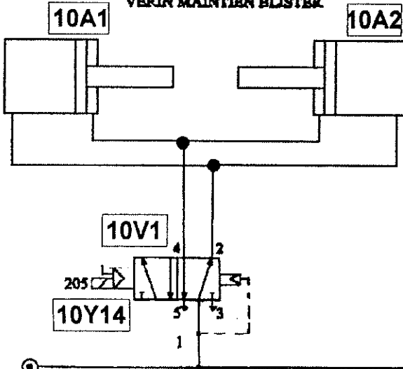
VERIN MAINTIEN BLISTER
